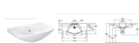
NADGRADNI LAVABO 65
